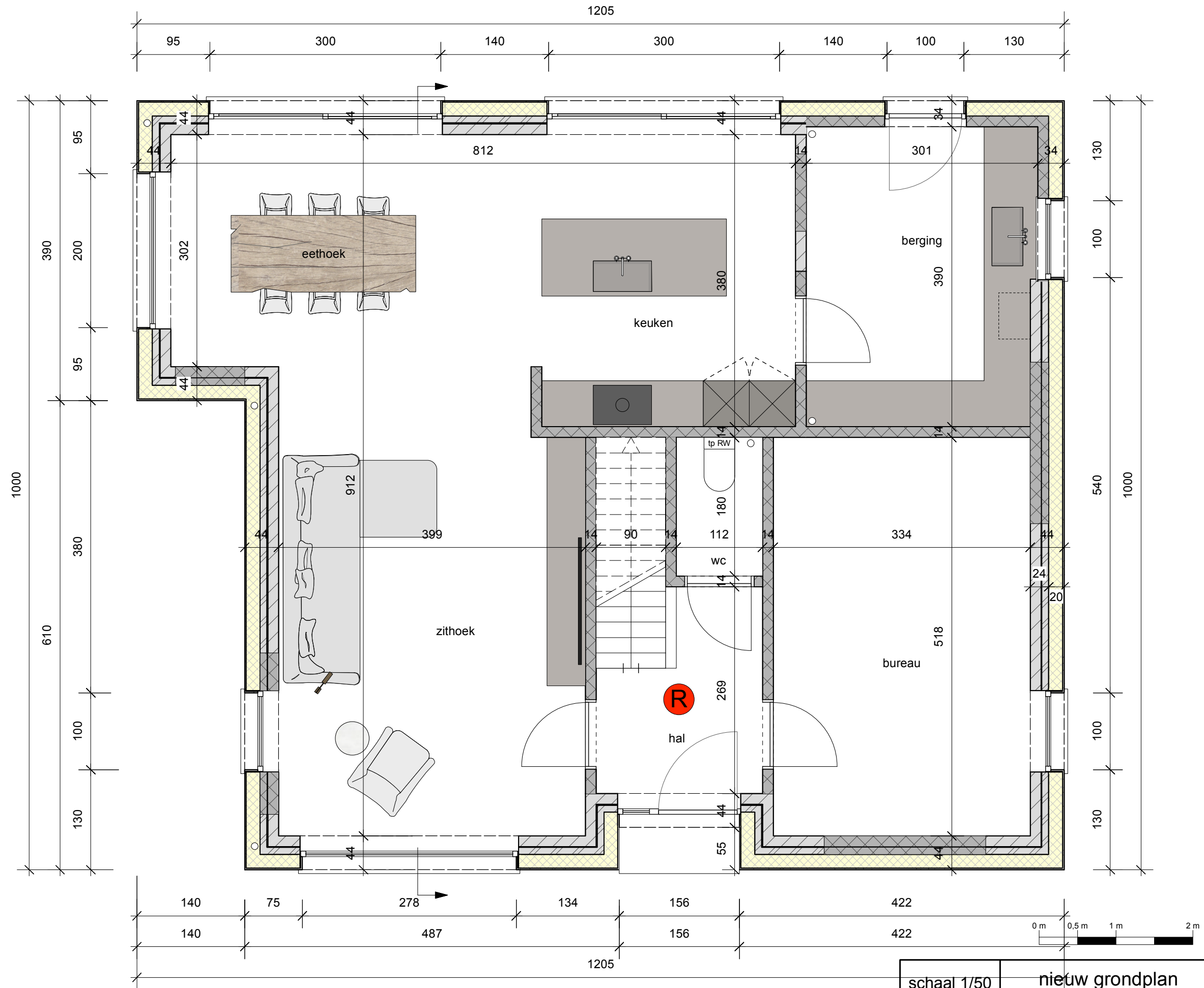
grondplan
