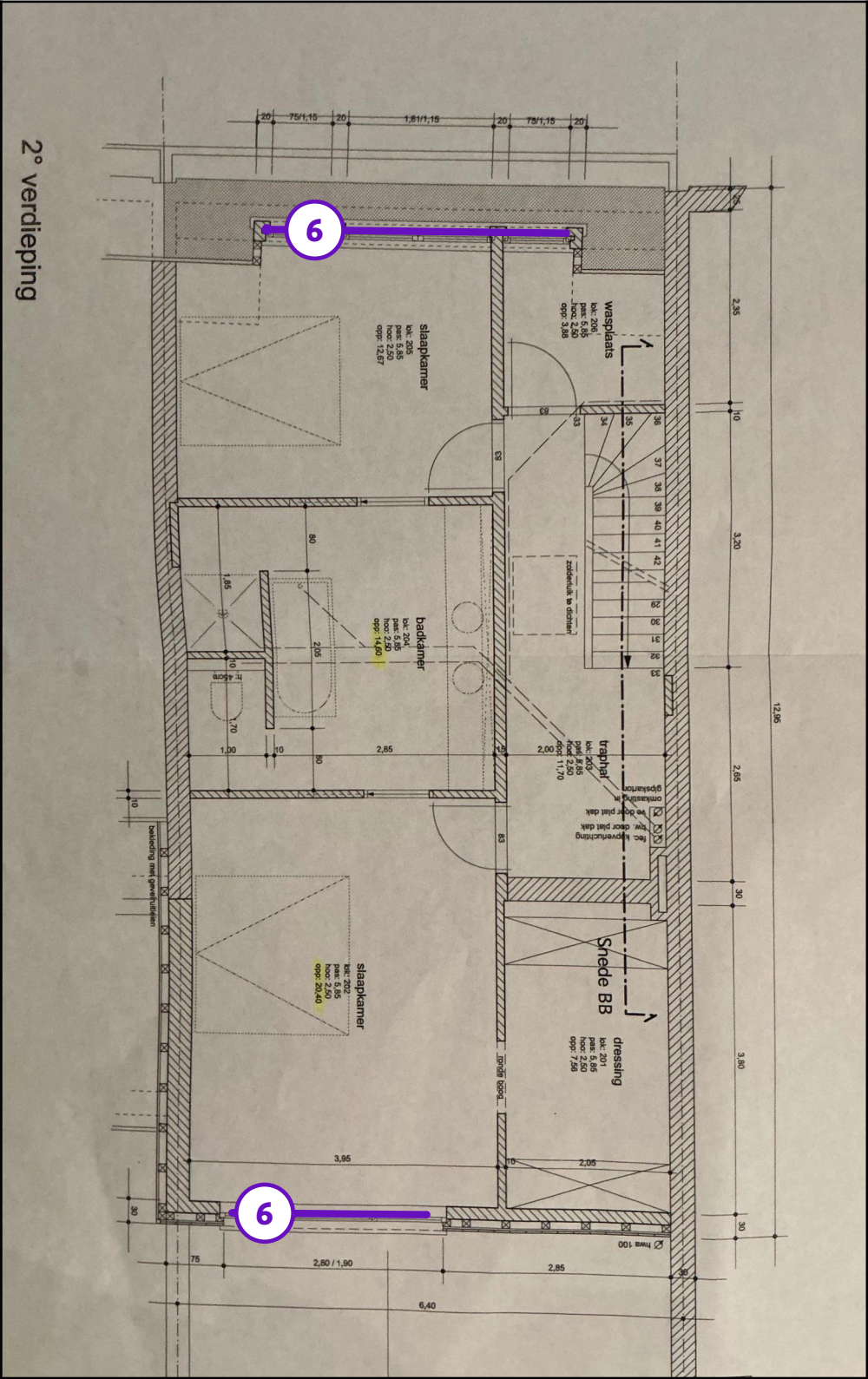
Legende van plan 1.6: 2de verdieping
