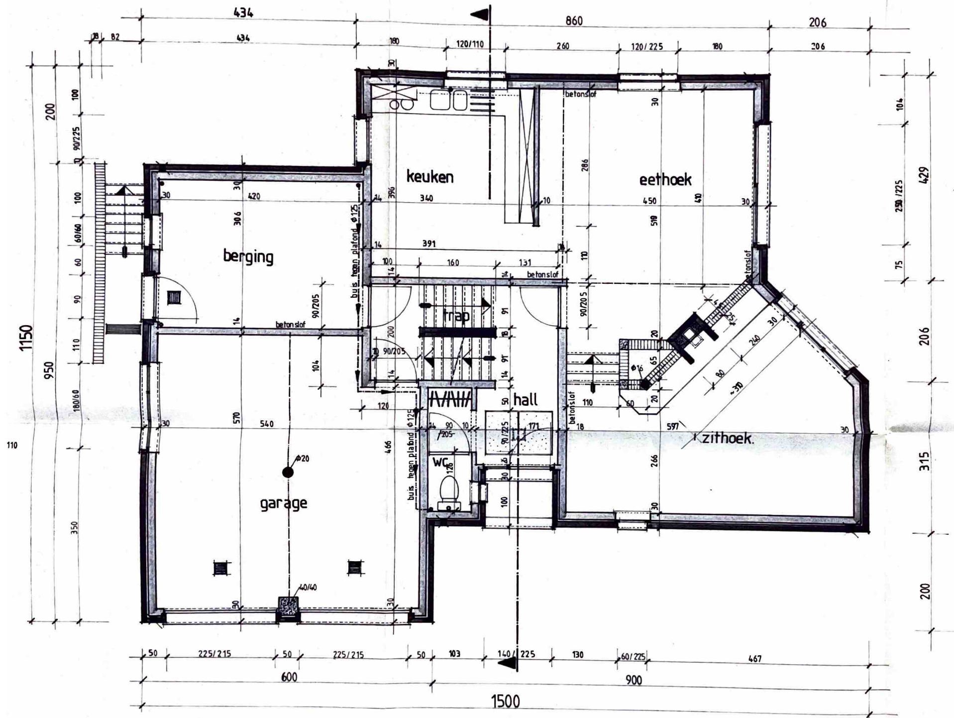
GRONDPLAN.
