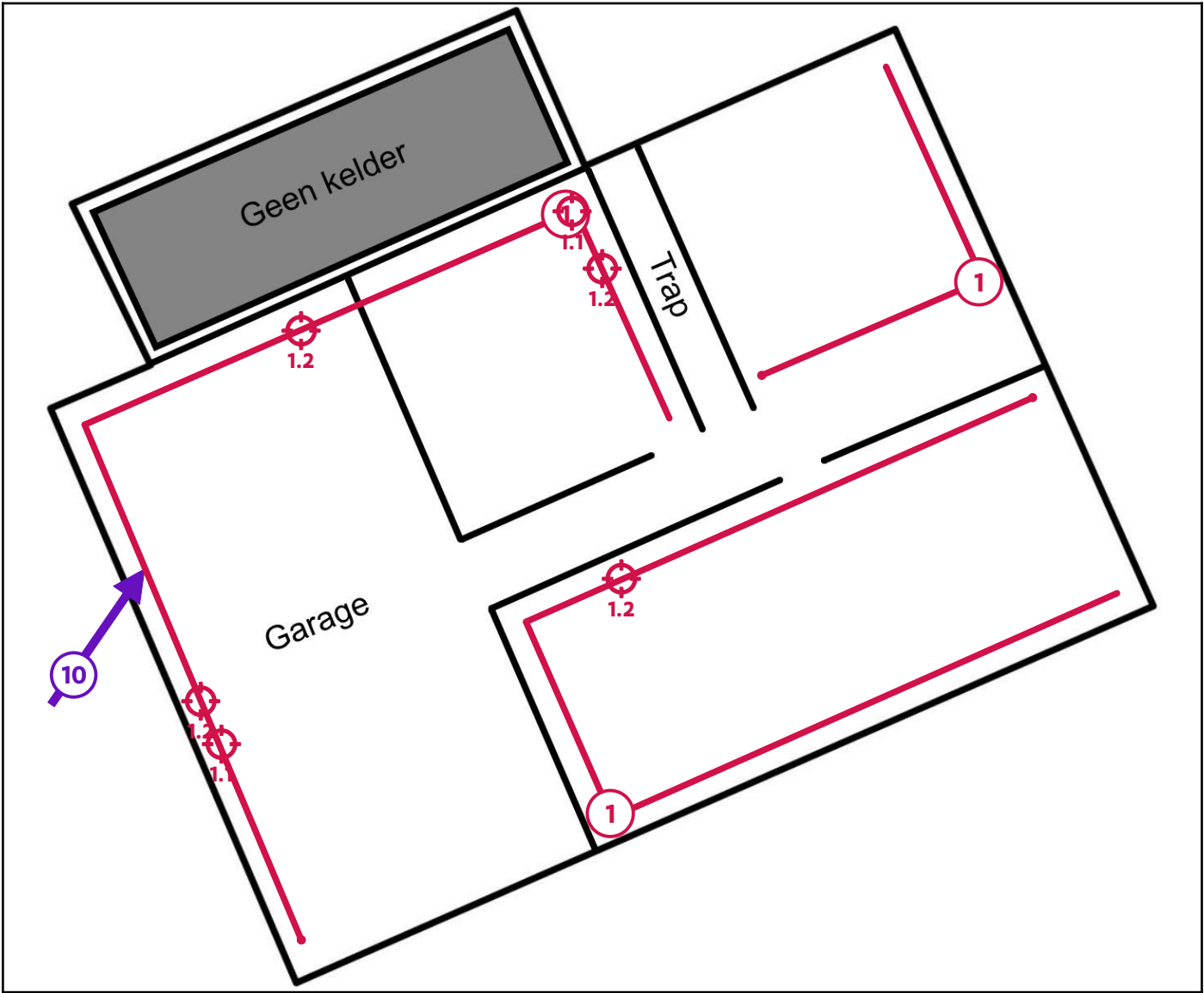
Legende van plan 1.3: Plan kelder
