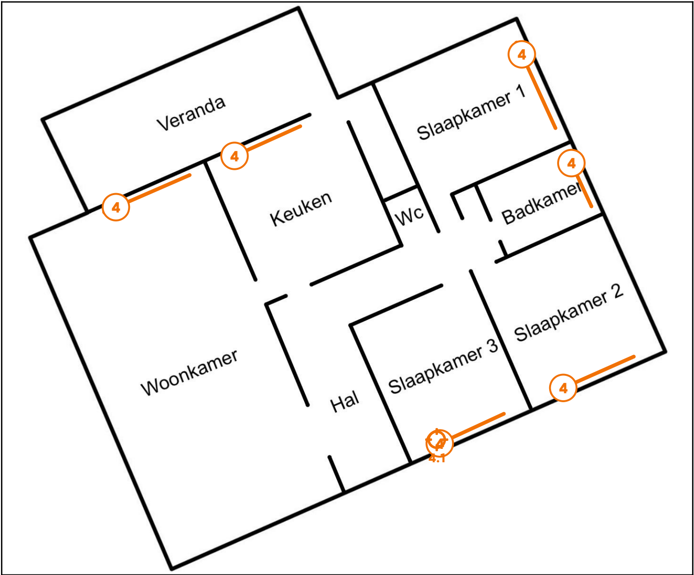
Legende van plan 1.6: Plan gelijkvloers (3)
