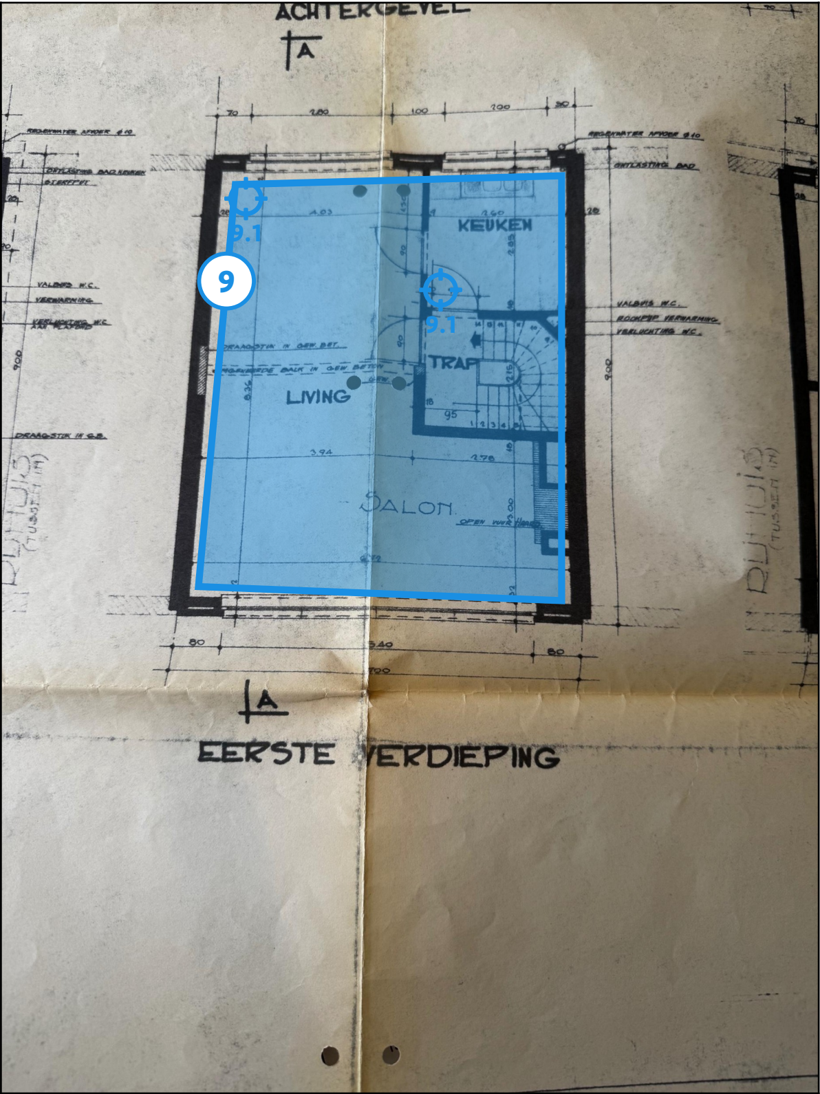
Legende van plan 1.5: Plan 1e verdiep (2)
