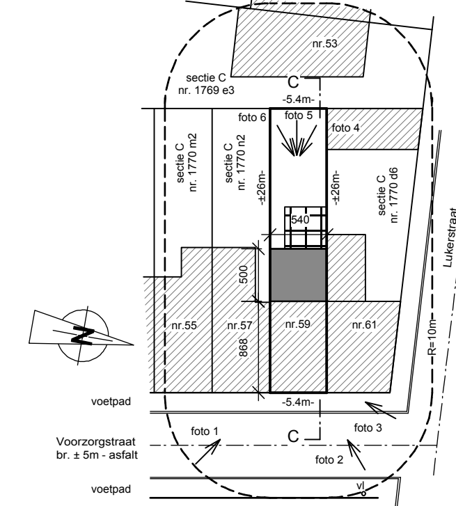
INPLANTINGSPLAN nieuwe toestand schaal 1/500
