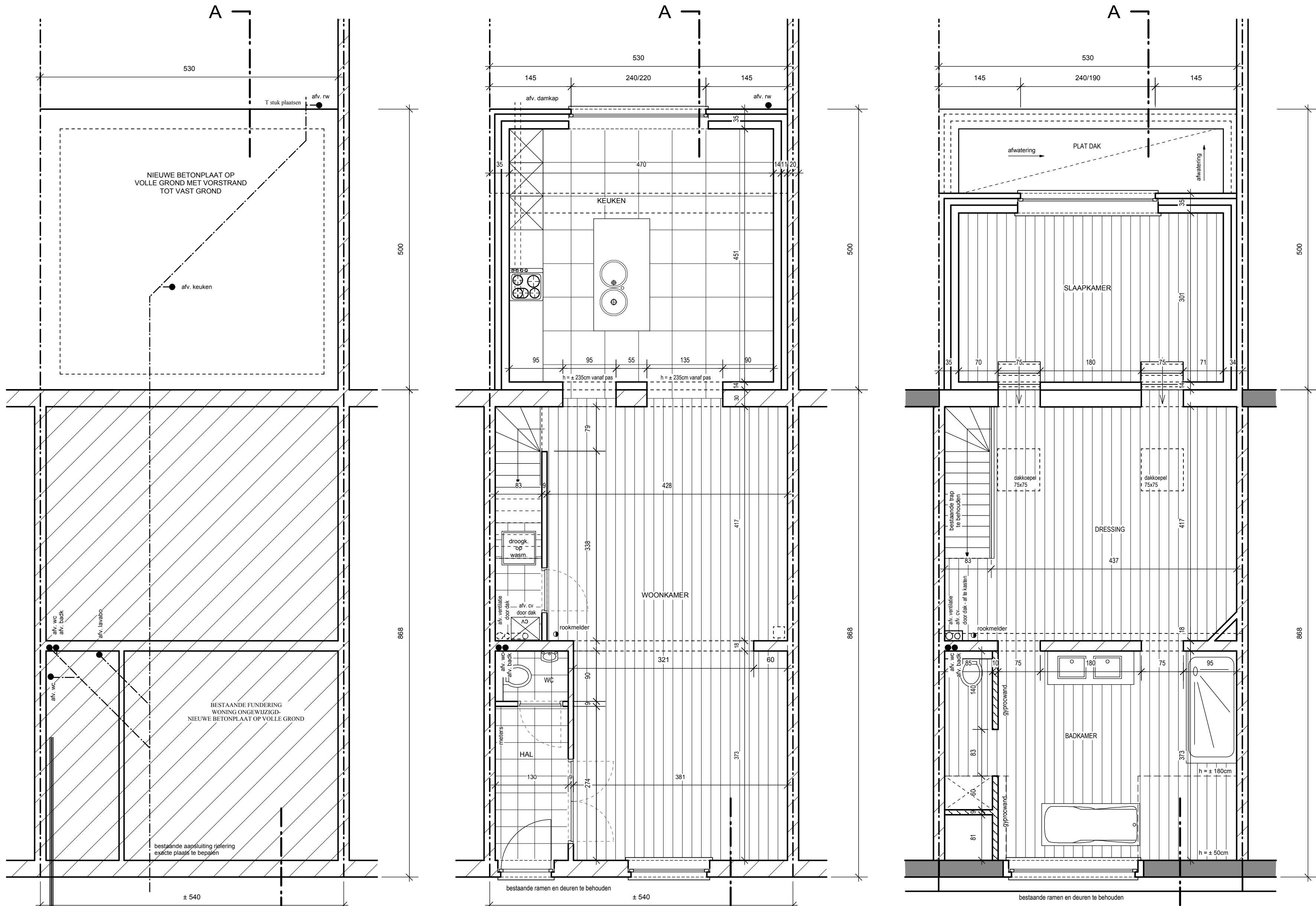
FUNDERINGS - EN RIOLERINGSPLAN
