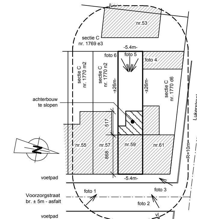
INPLANTINGSPLAN bestaande toestand schaal 1/500
