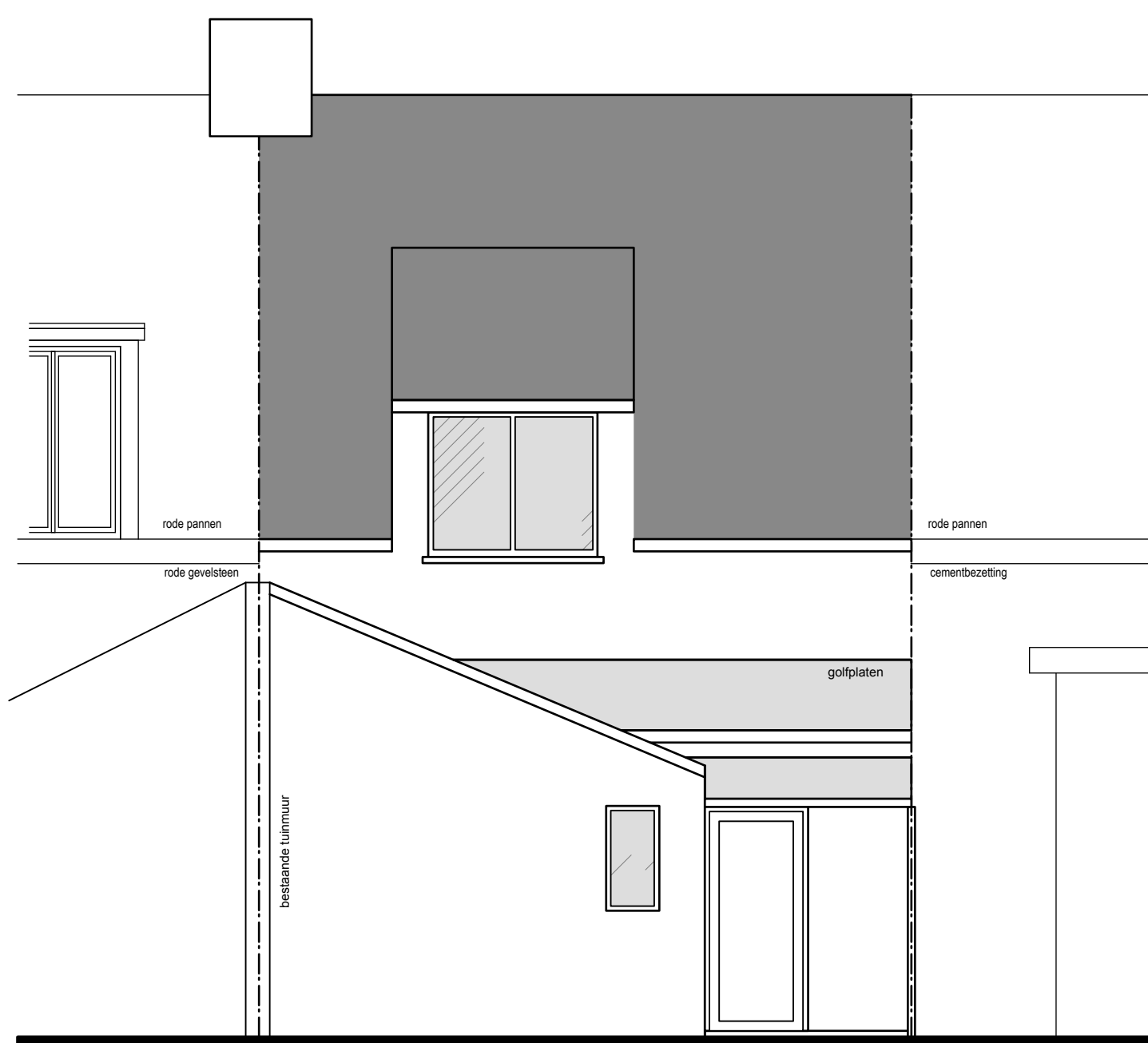
ACHTERGEVEL bestaande toestand
