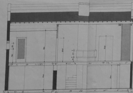
COUPE AA
