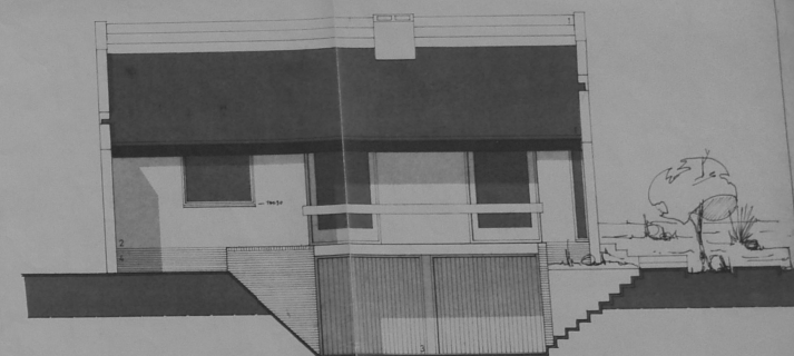
FACADE PRINCIPALE
