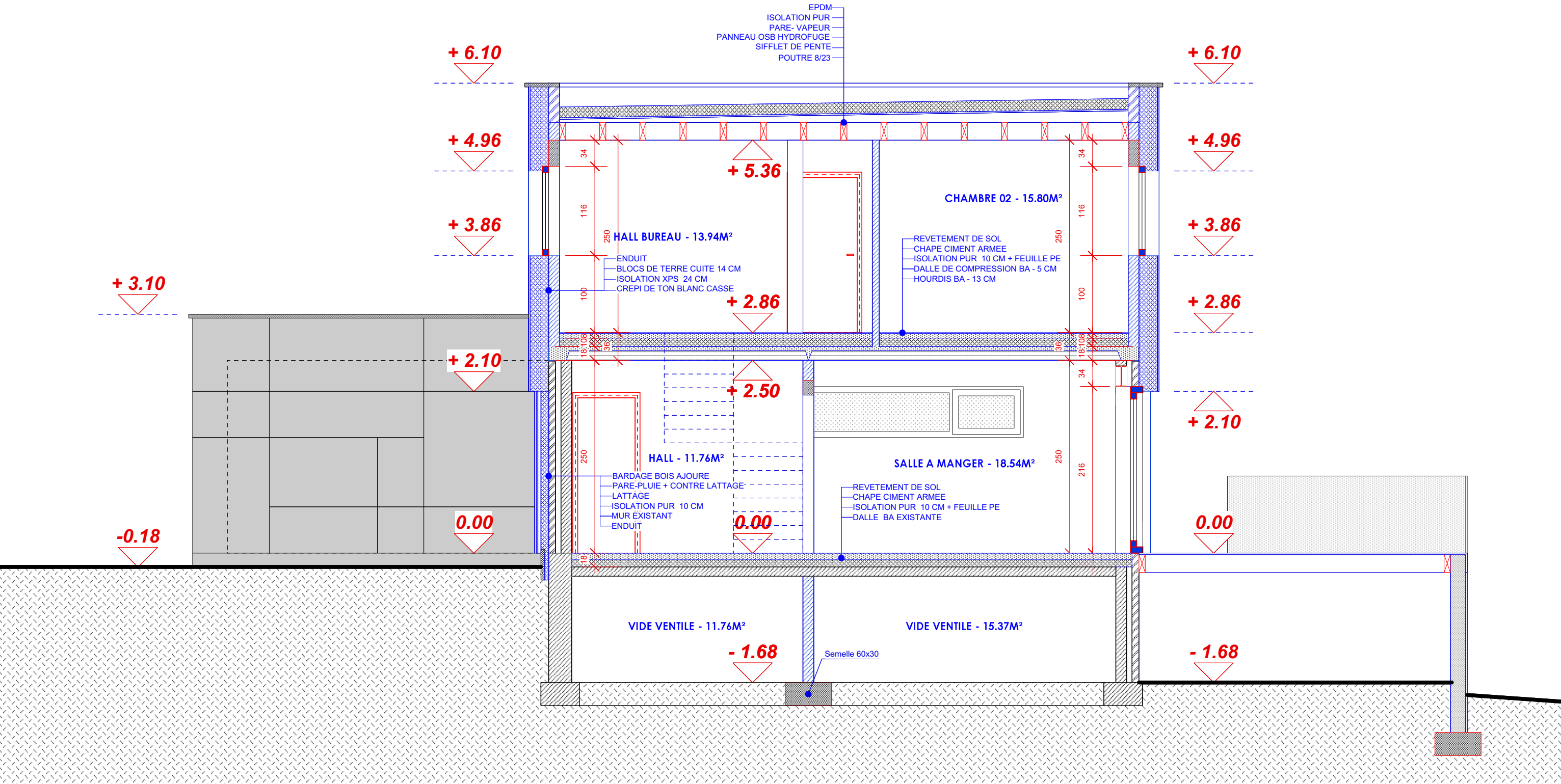
COUPE AA
