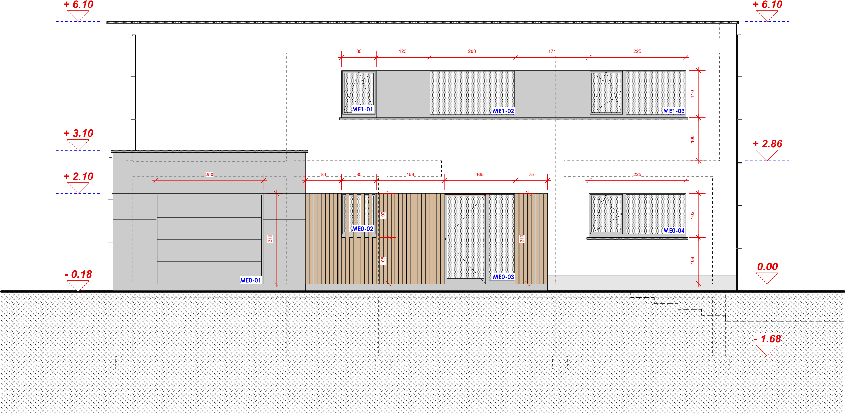
FACADE AVANT
