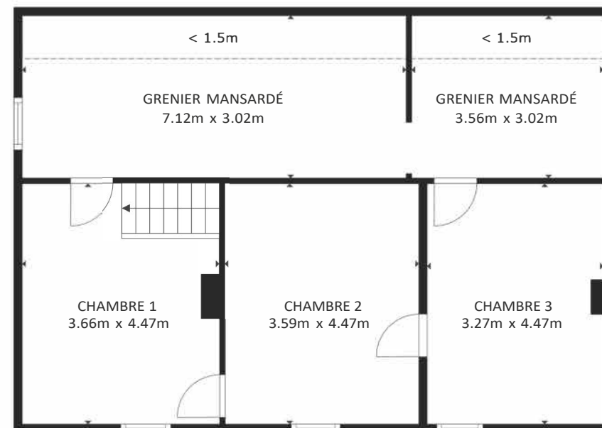
1er ETAGE
