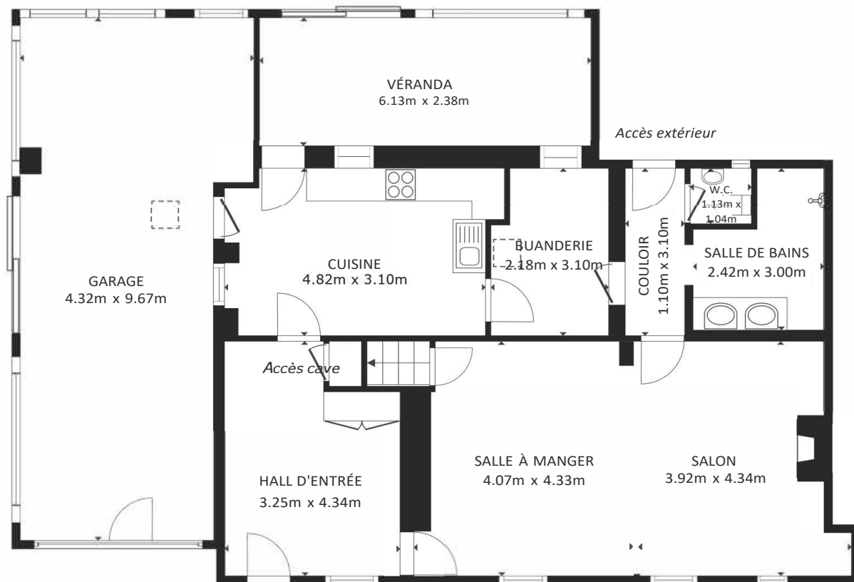
REZ-DE-CHAUSSEE
