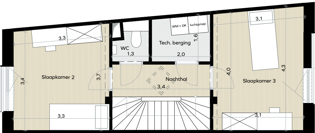
niv +2
