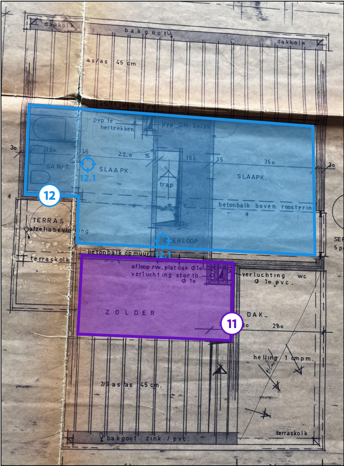
Legende van plan 1.7: Verdiep 1 - Plafond
