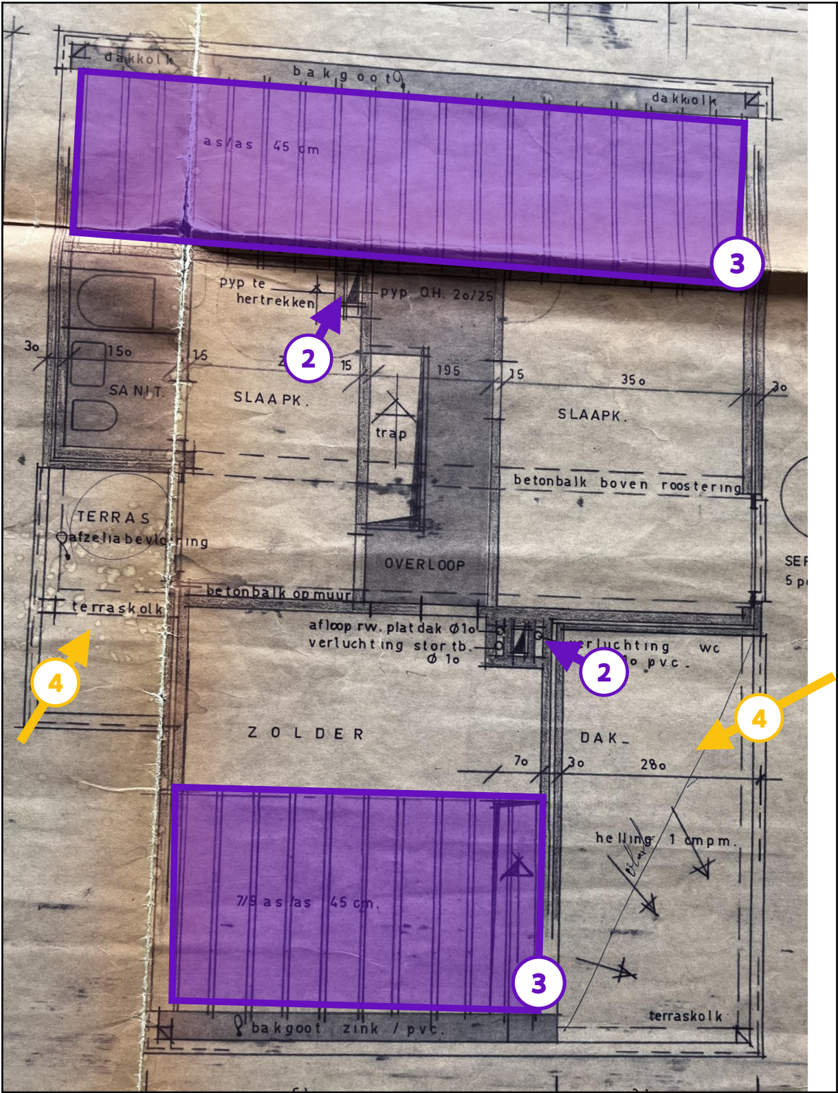
Legende van plan 1.10: Beperking dak/onderdak
