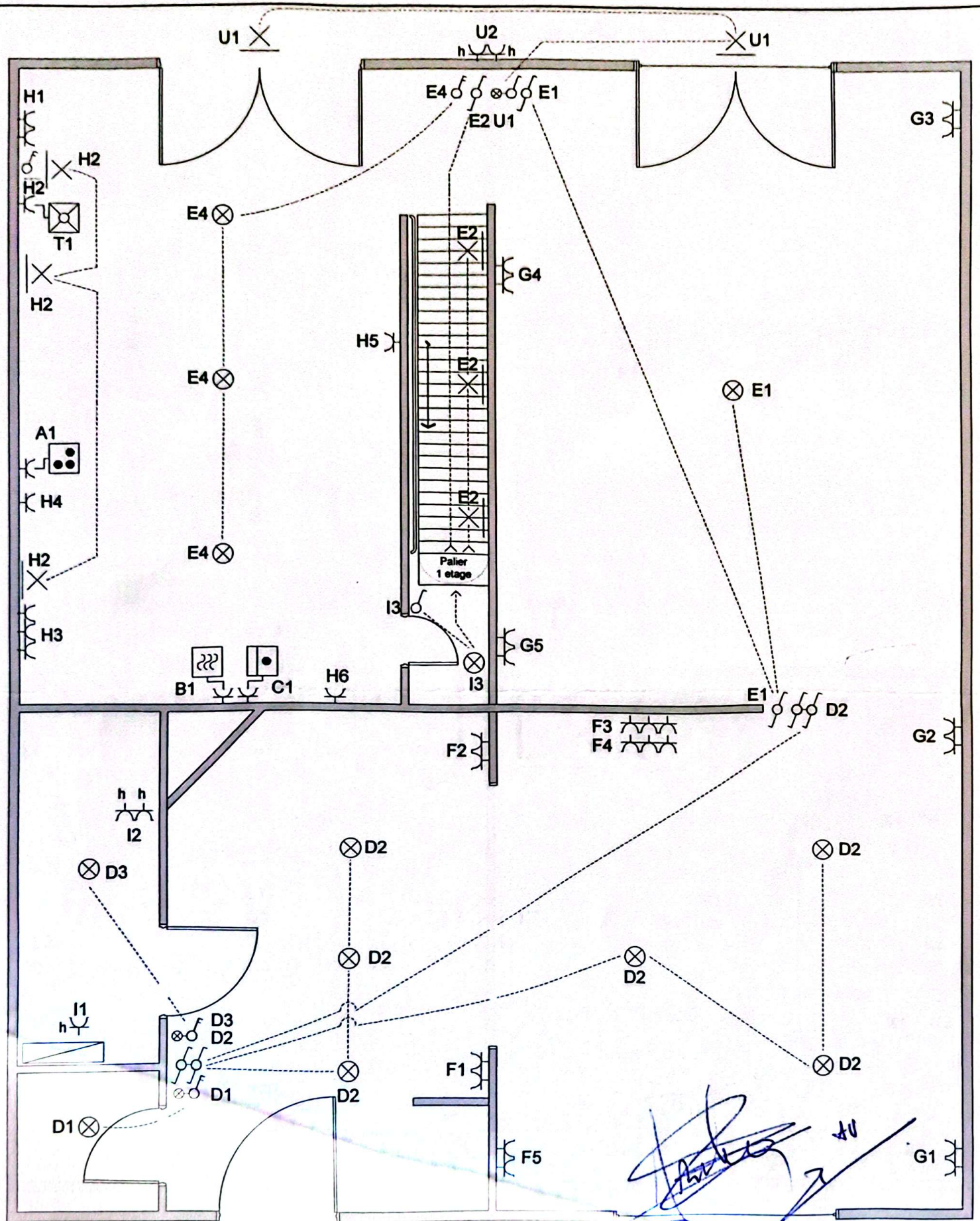
Schéma de position Rez-de-chausée
