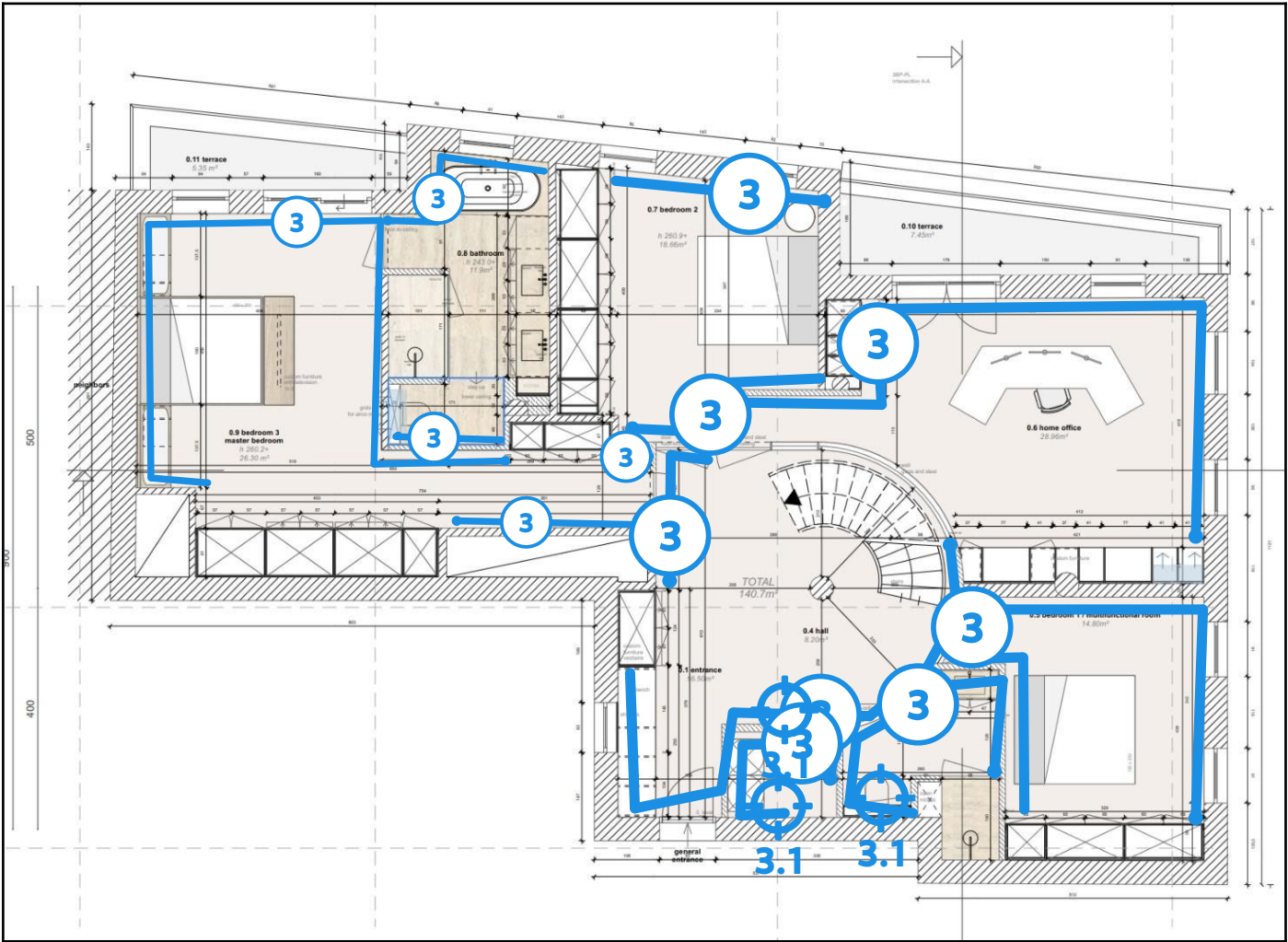
Legende van plan 1.1: Duplex - gelijkvloers
