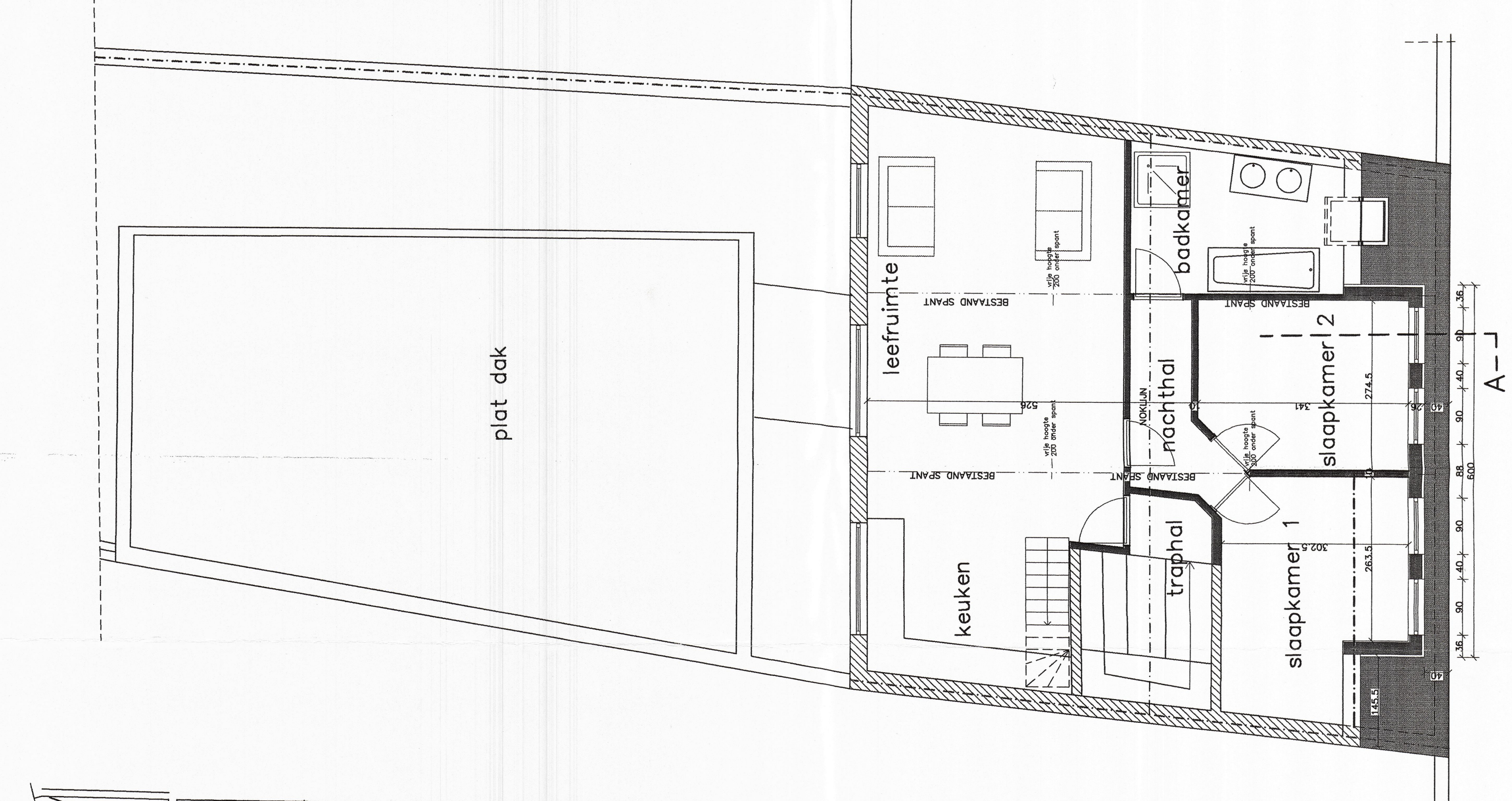
GRONDPLAN VERDIEPING bestaande toestand SCHAAL 1/100
