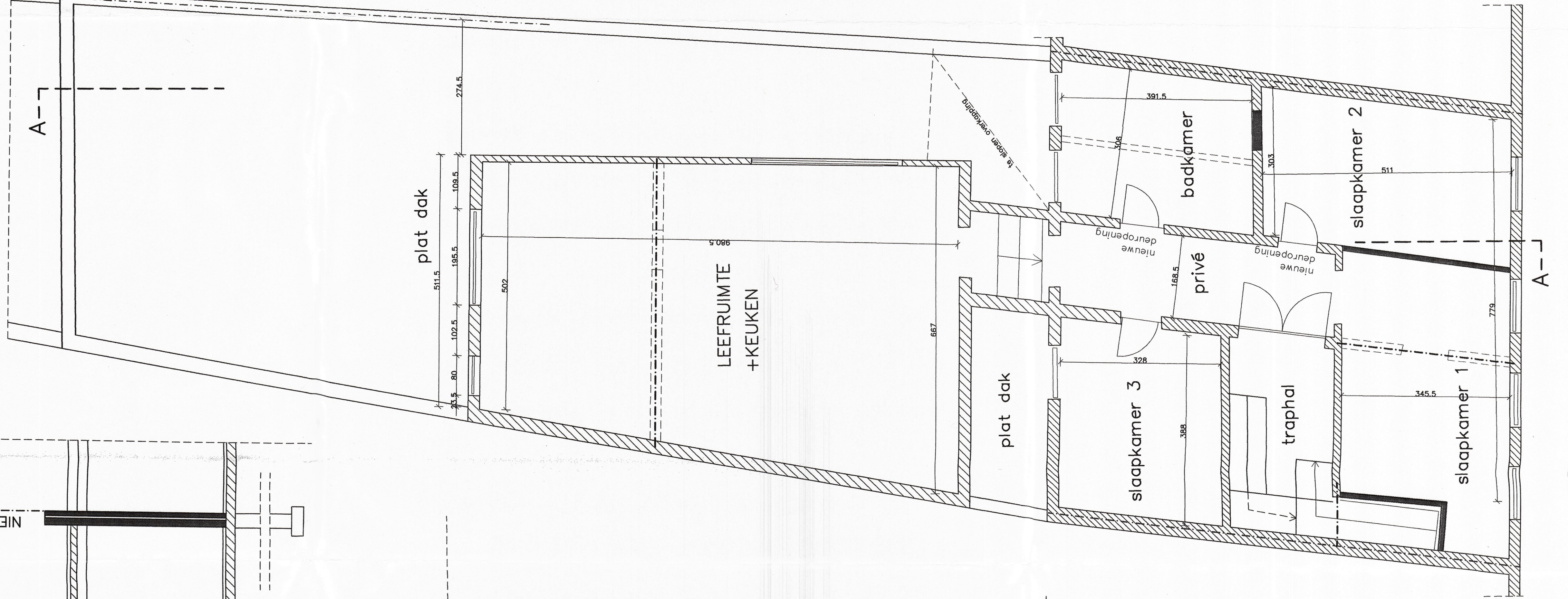
GRONDPLAN VERDIEPING bestaande toestand SCHAAL 1/100
