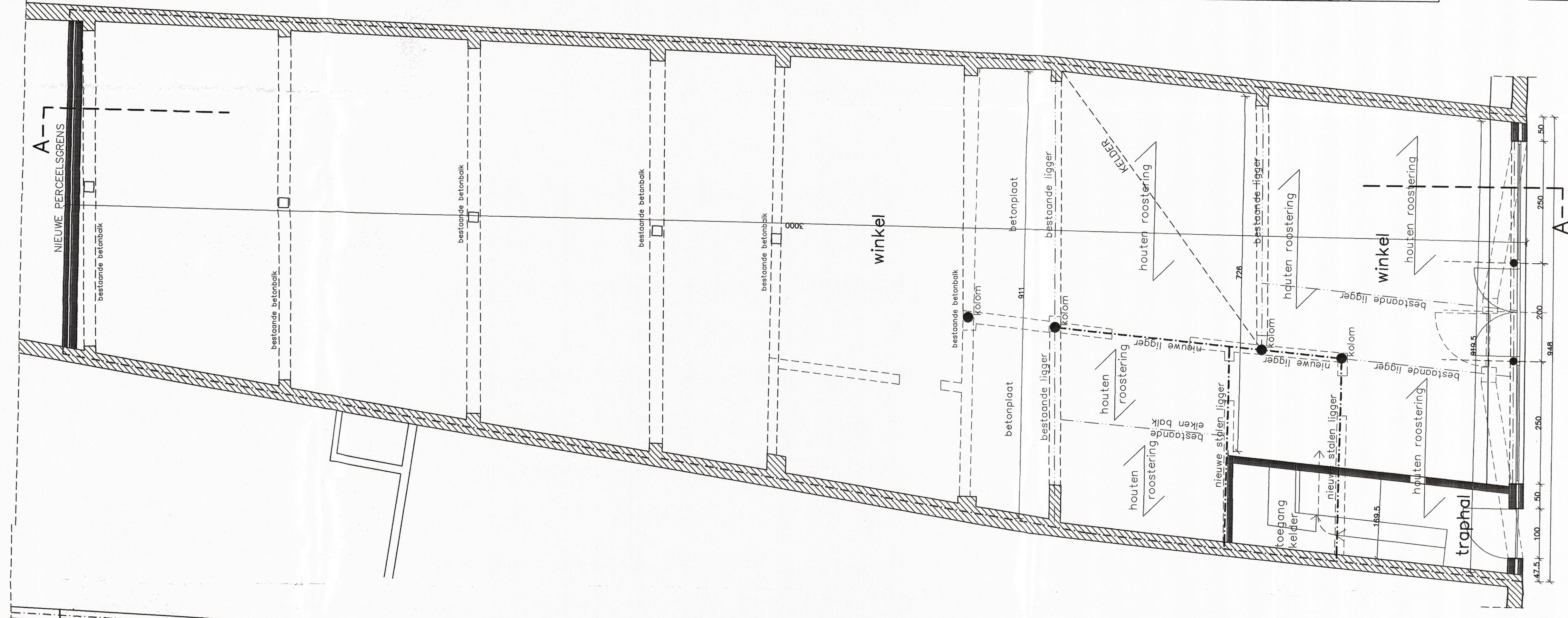
GRONDPLAN VERDIEPING bestaande toestand SCHAAL 1/100
