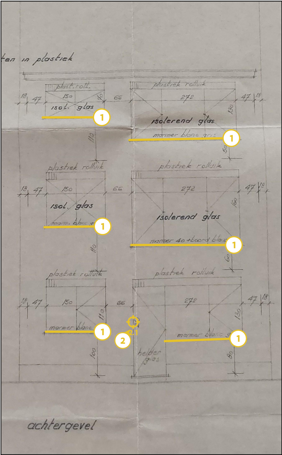
Legende van plan 1.12: Achtergevel
