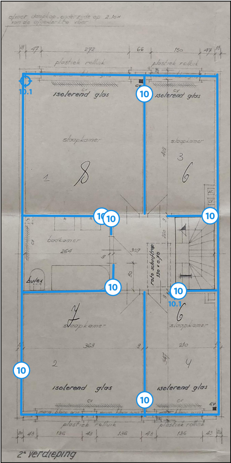
Legende van plan 1.8: 2e verdieping
