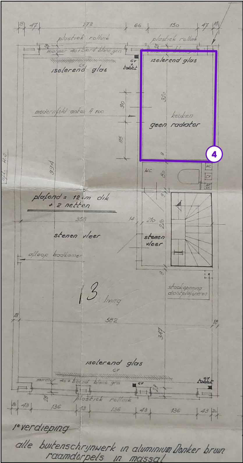
Legende van plan 1.13: Verdieping 1
