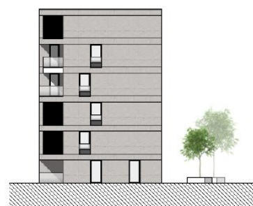
ZIJGEVEL
