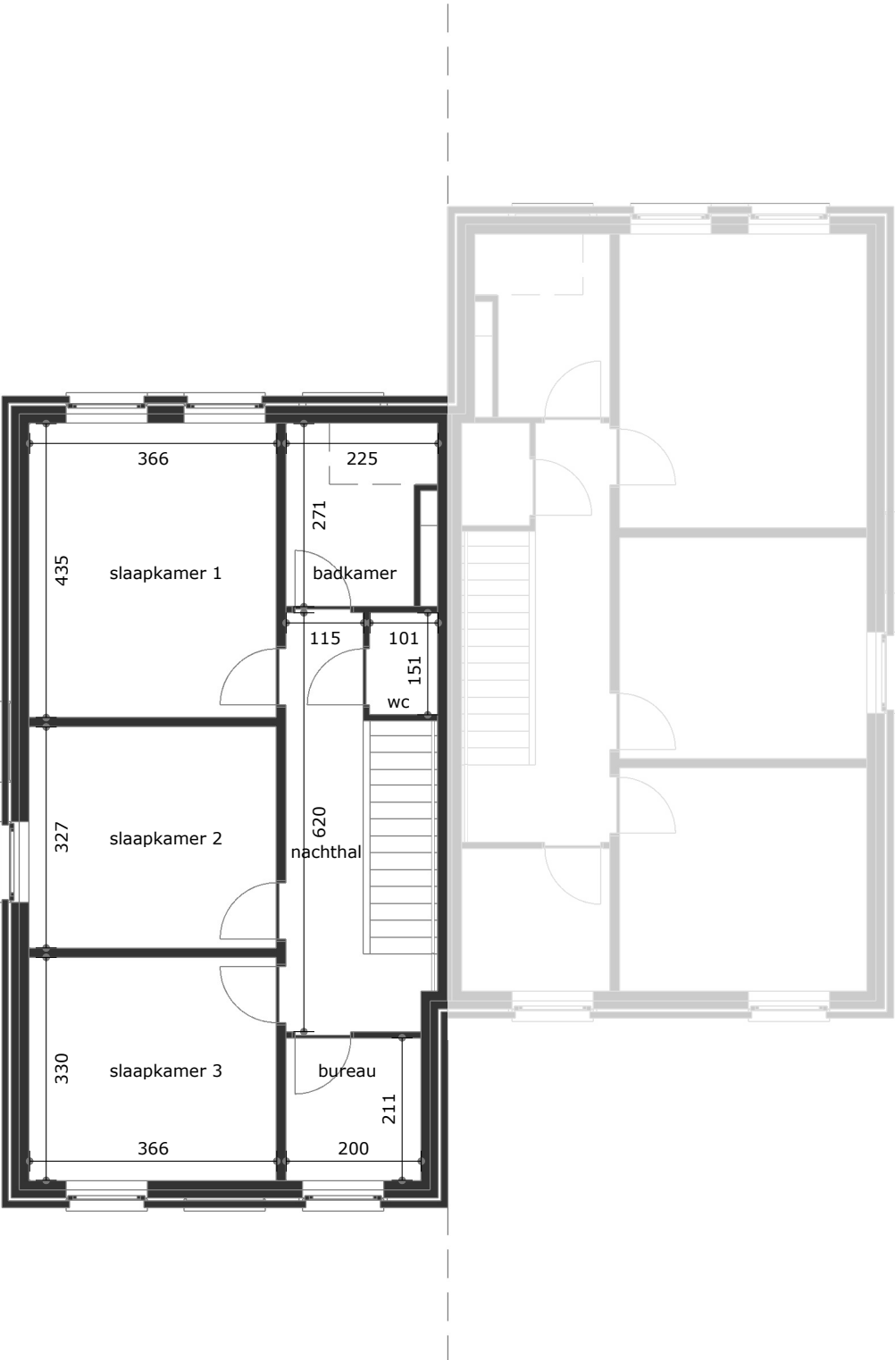
VERDIEPING
