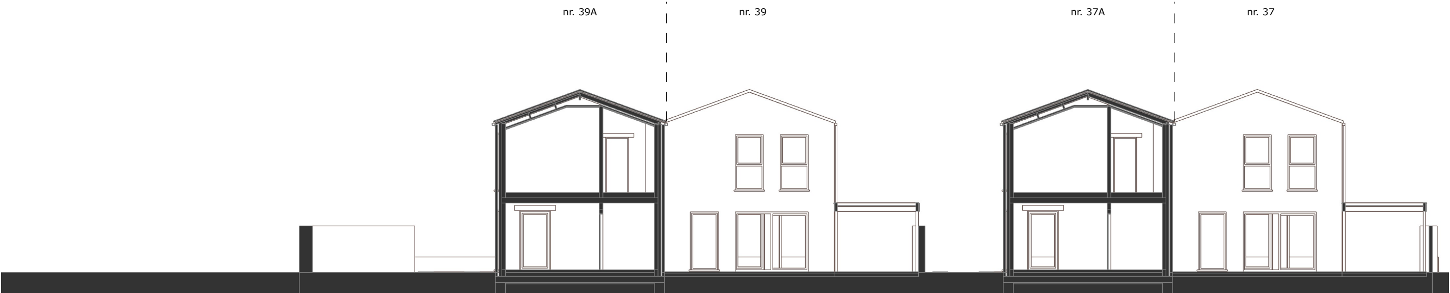
SNEDE BB
