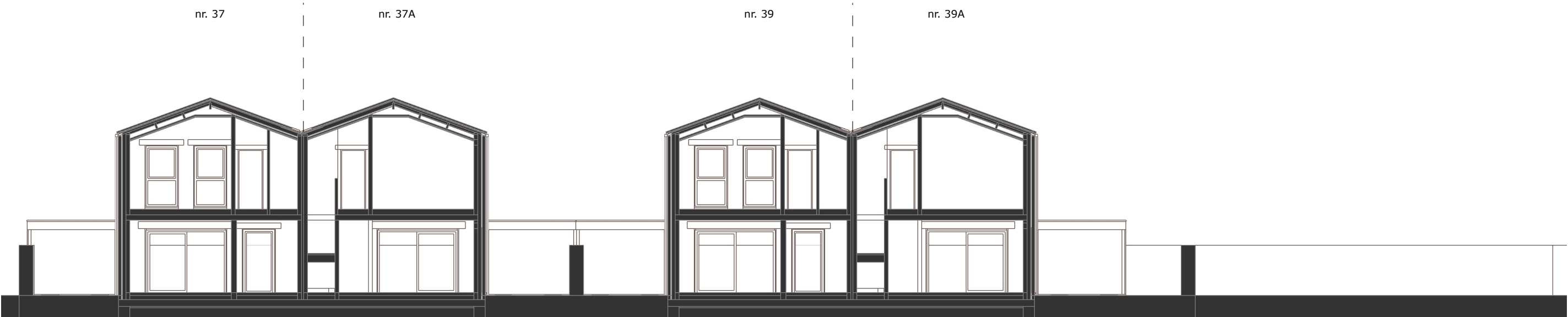
SNEDE AA
