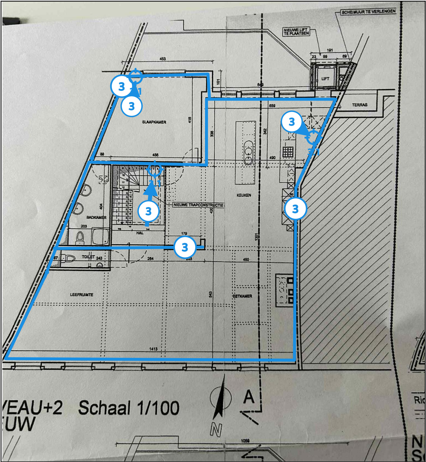
Legende van plan 1.1: 2e verdieping
