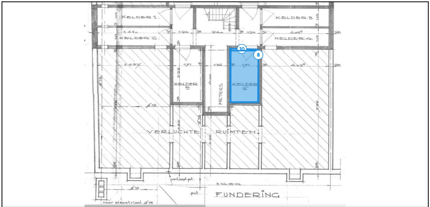
Legende van plan 1.4: Plan kelderverdieping
