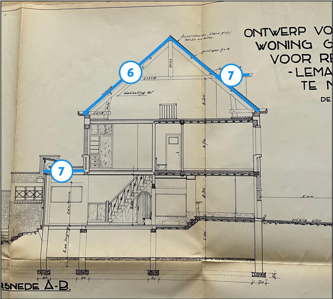
Legende van plan 1.4: Doorsnede
