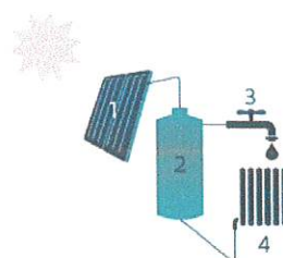
1. Zonnecollector | 2. Opslagvat 3. Koudwater toevoer 4. Warmwater afvoer
