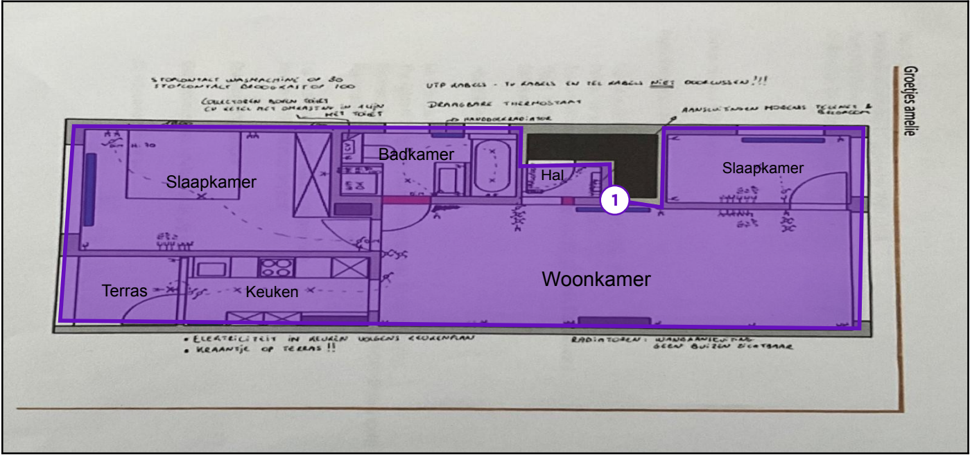
Legende van plan 1.3: Ondervloeren / restanten oude lijmlagen
