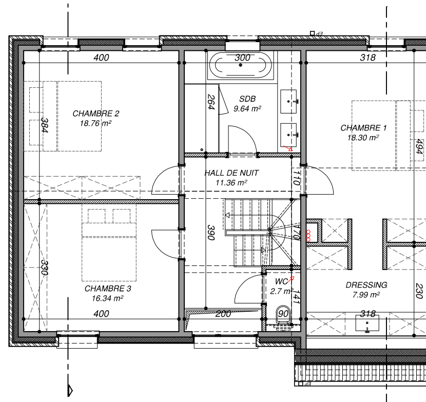
Plan ETAGE
