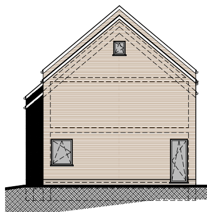
Façade LATÉRALE
