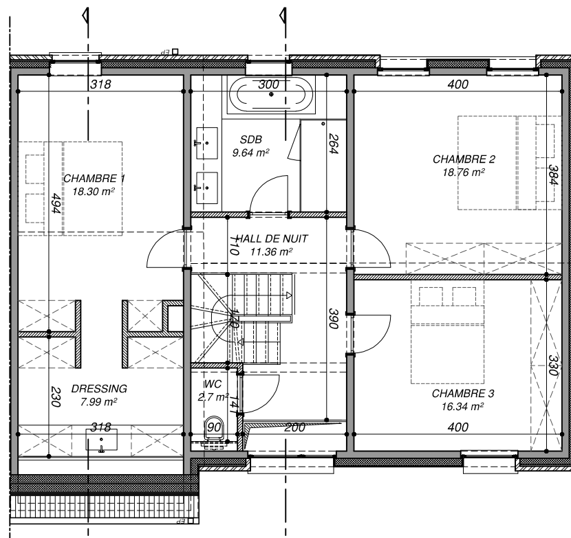
Plan 1ER ÉTAGE
