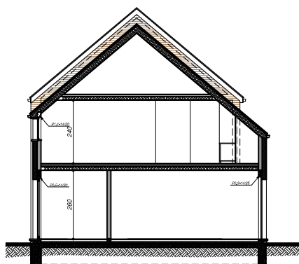
Coupe
