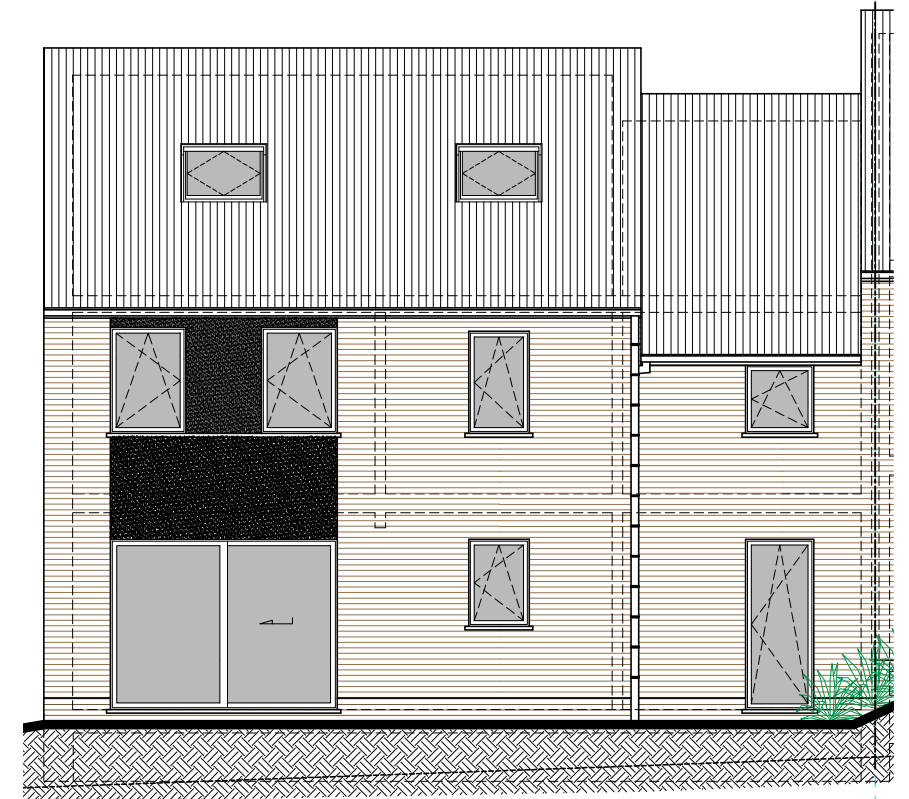
Façade ARRIÈRE
