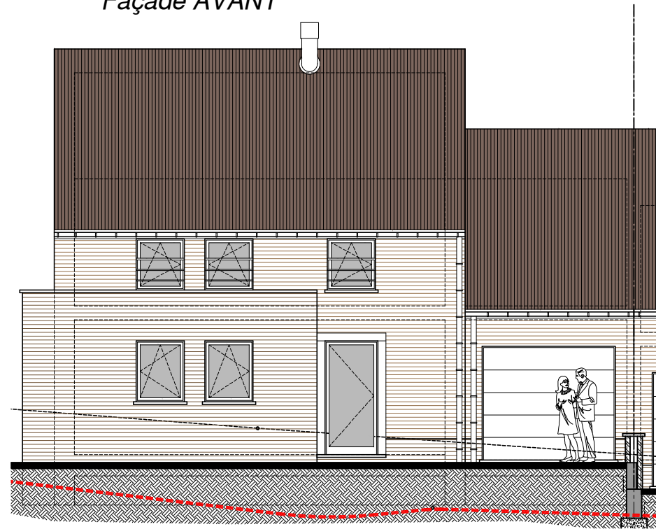
Façade AVANT
