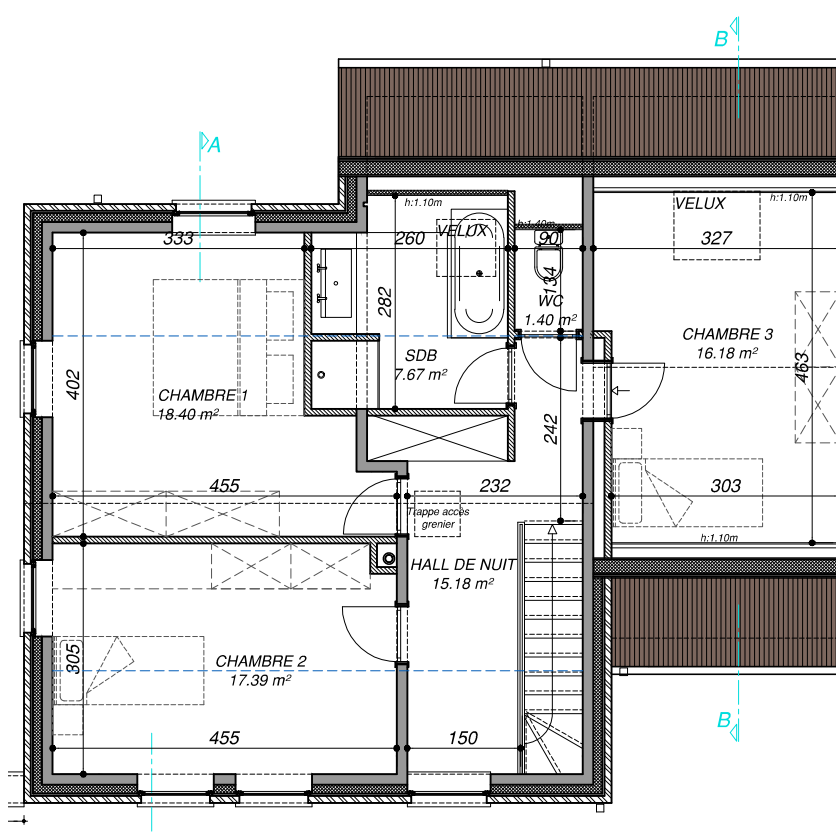
Plan ETAGE
