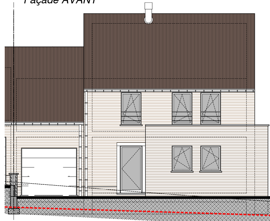
Façade AVANT
