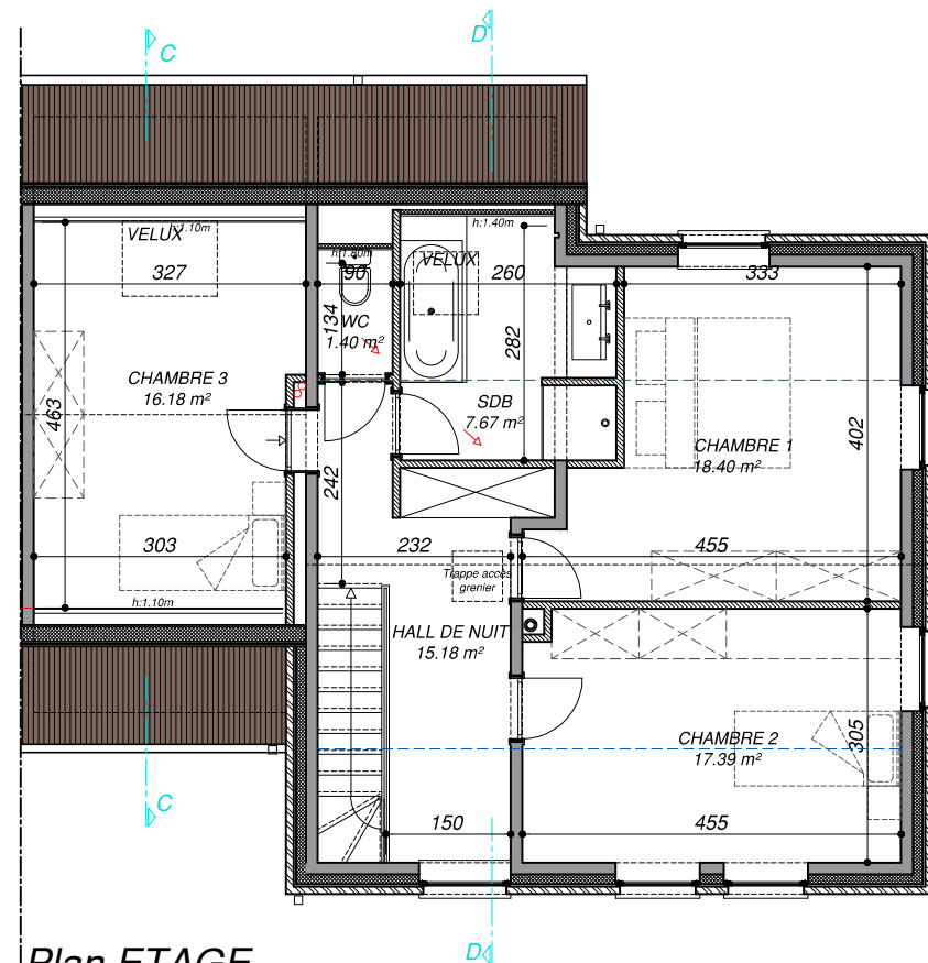
Plan ETAGE
