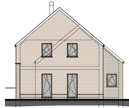
Façade LATÉRALE
