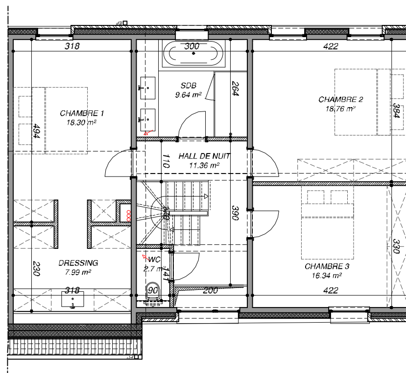
Plan ETAGE
