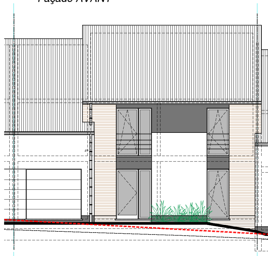
Façade AVANT
