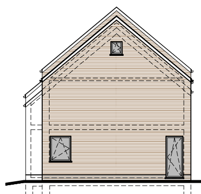
Façade LATÉRALE
