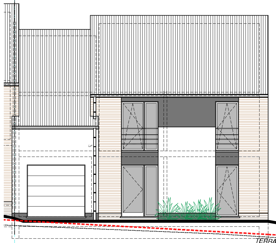
Façade AVANT
