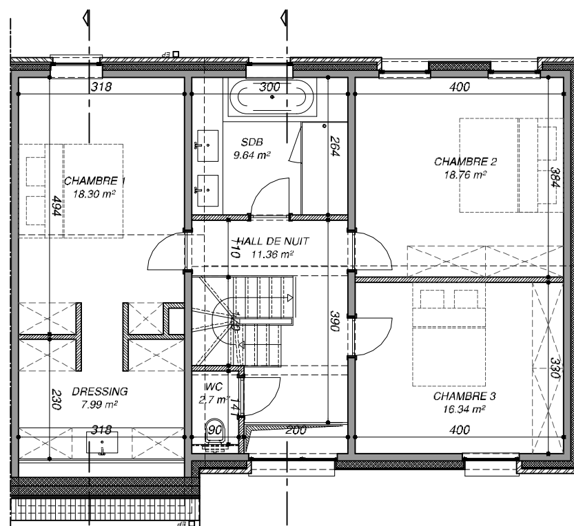
Plan 1ER ETAGE
