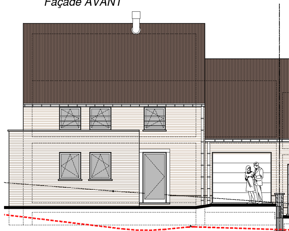
Façade AVANT
