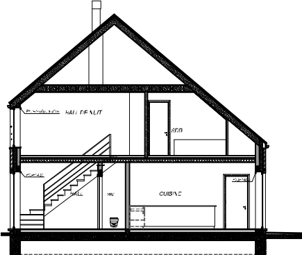
Coupe
