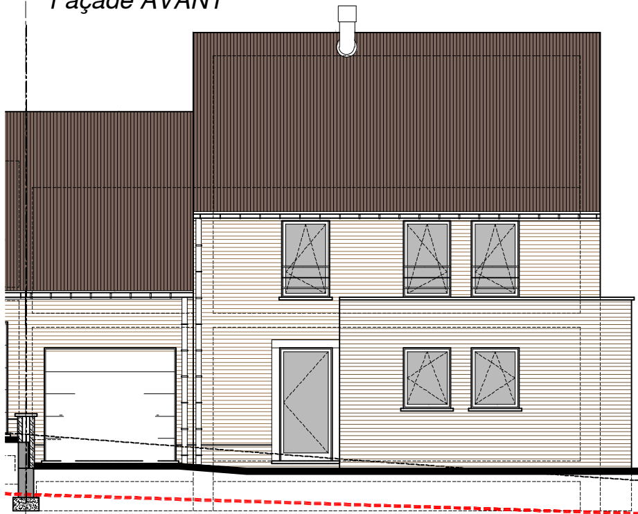
Façade AVANT
