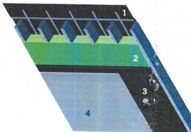
1. Onderdak | 2. Isolatie | 3. Dampscherm | 4. binnenaftrekking
