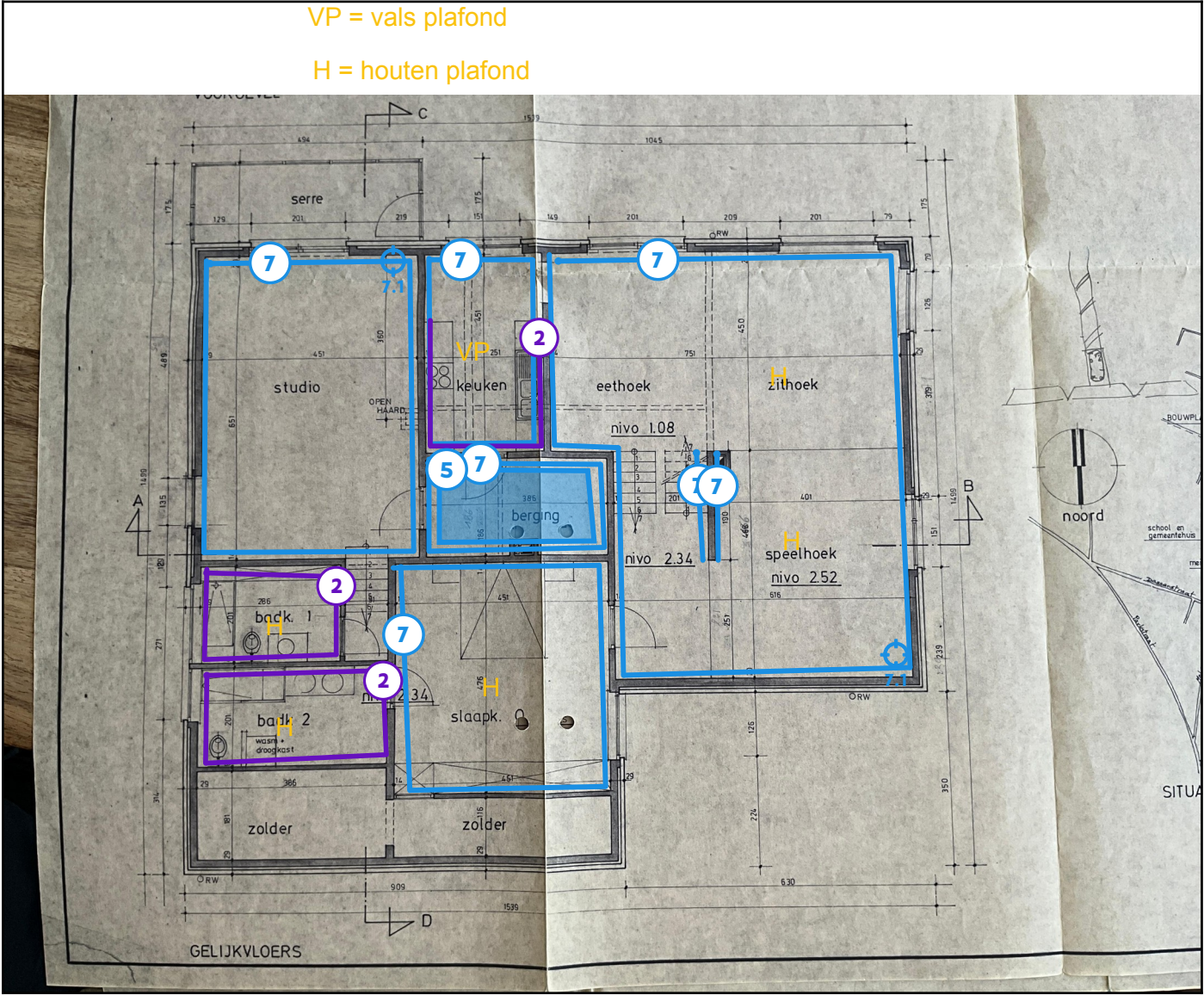
Legende van plan 1.4: gelijkvloers en tussenverdieping
