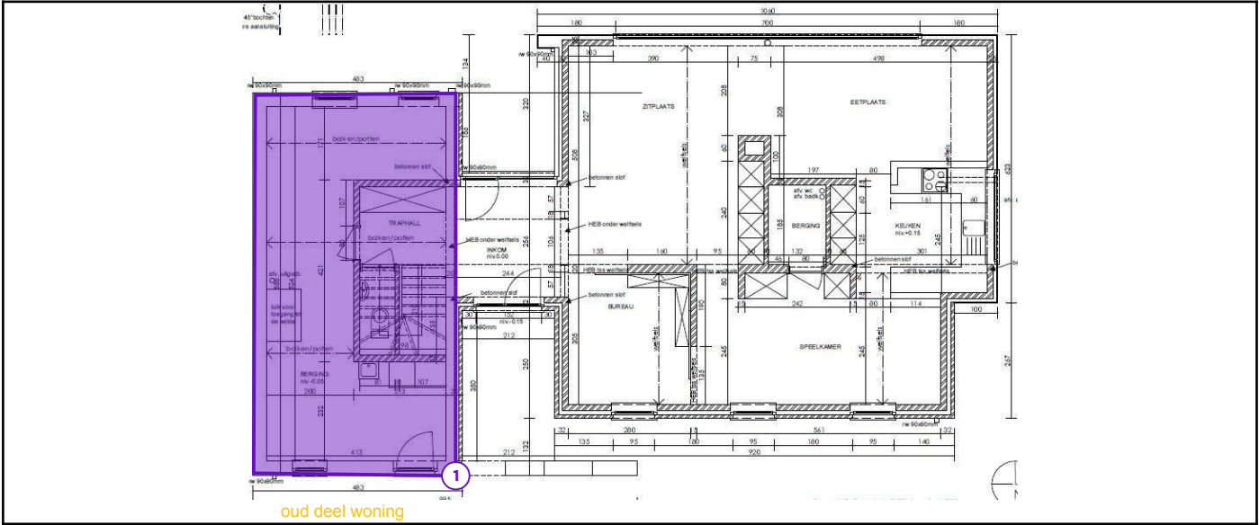
Legende van plan 1.3: Gelijkvloers
