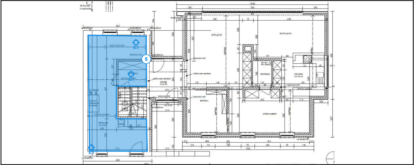
Legende van plan 1.4: Gelijkvloers
