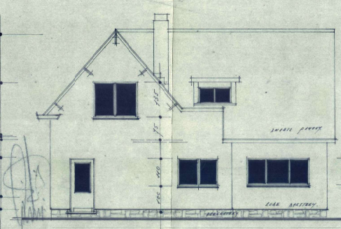
ACHTERGEVEL
