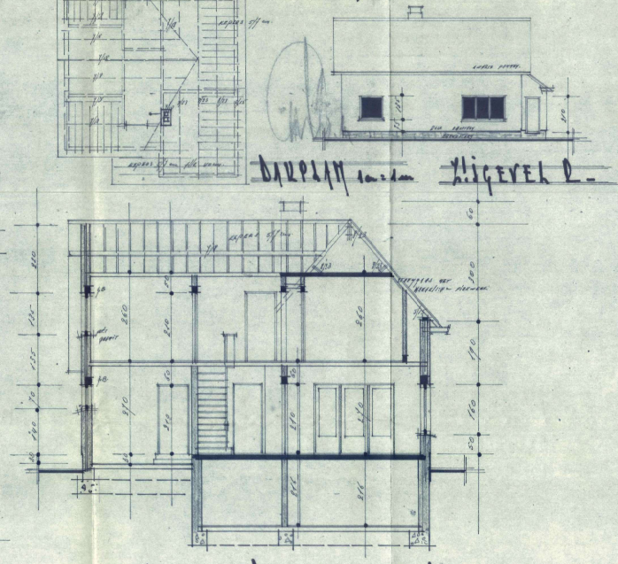
DOORSNIJDE A-A
