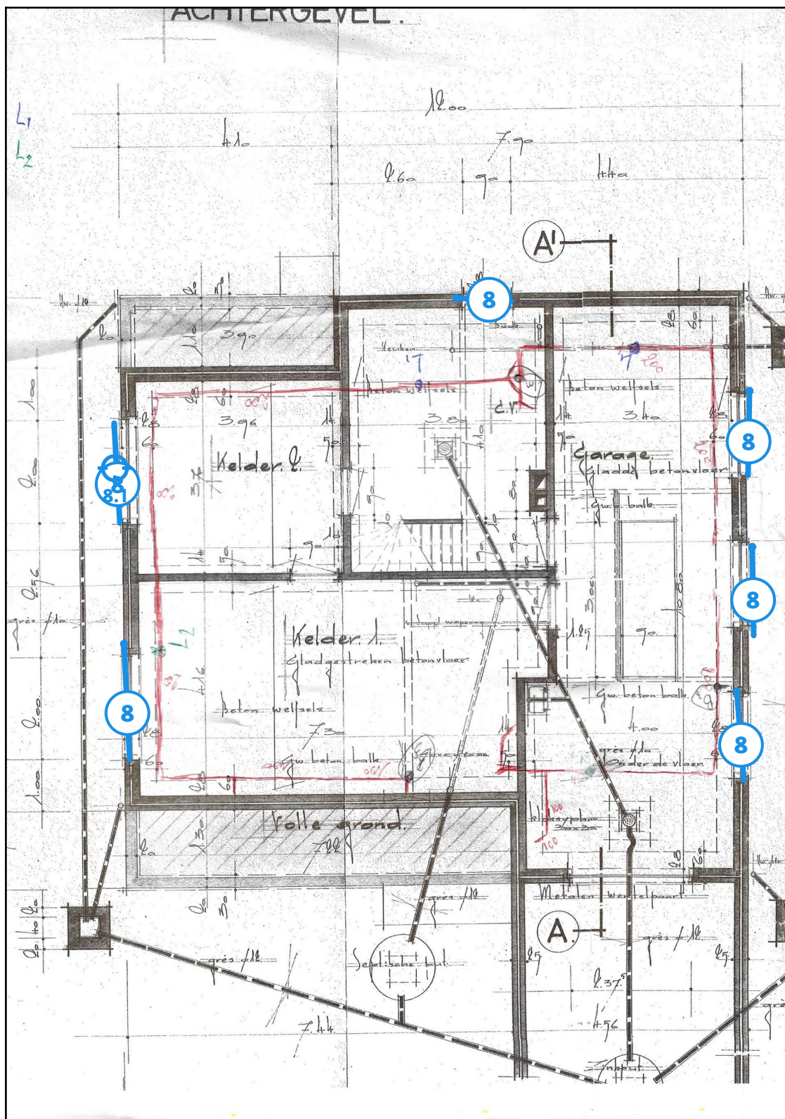
Legende van plan 1.2: kelderplan
